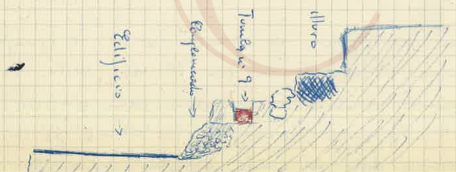
Esquema sección N-5
