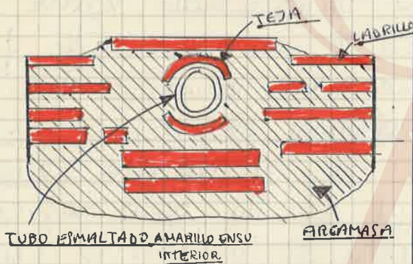
CROQUIS DE LA CLOACA MODERNA
